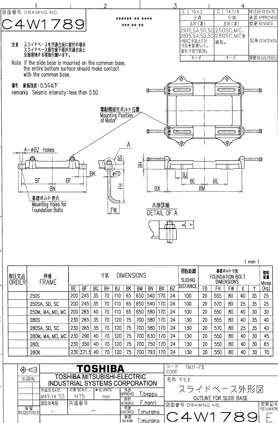
図1 スライドベース外形図 (枠番 250・280)
